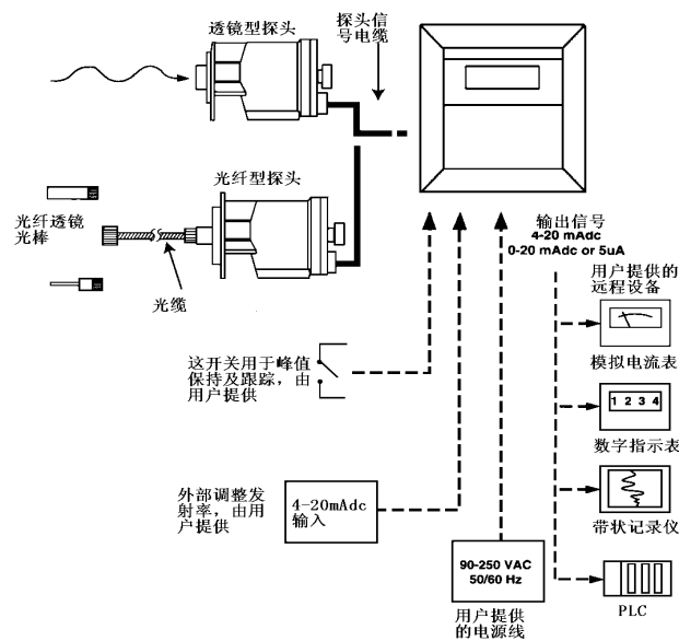
Mirage 透镜型和光纤型系统的配置
